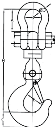
20t -30t [アイフック]
